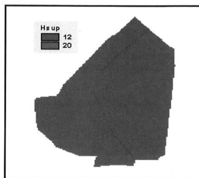
Imagen 19. Hidrología superficial.
