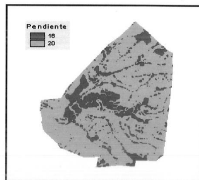
Imagen 23. Pendiente.
