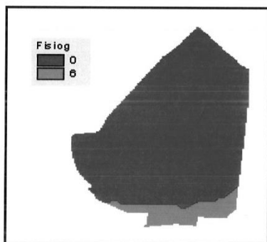
Imagen 16. Fisiografía.
