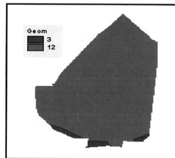
Imagen 15. Geomorfología
