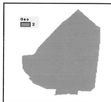
Imagen 17. Geología.
