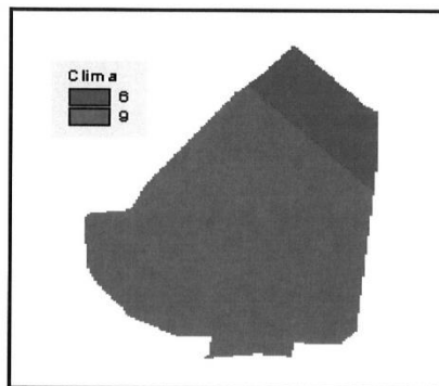
Imagen 18. Clima.
