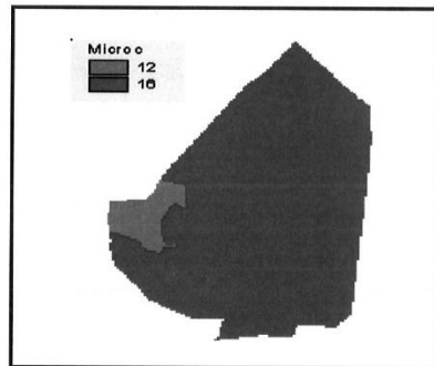
Imagen 14. Microcuencas.
