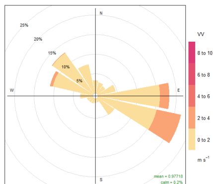
Gráfica 11. Rosa de vientos de la estación Félix Osoreo (FEO). Noviembre 2024.
