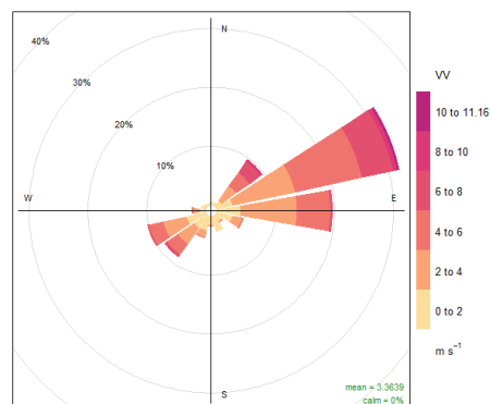
Gráfica 12. Rosa de vientos de la estación Epigmenio González (EPG). Noviembre 2024.
